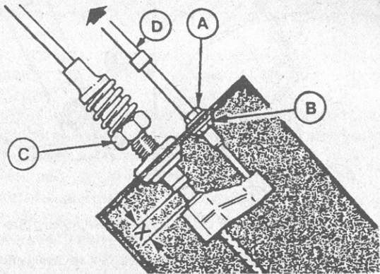
Рис. 11.14. Регулировка троса механизма kick-down в 1-ой версии исполнения.
