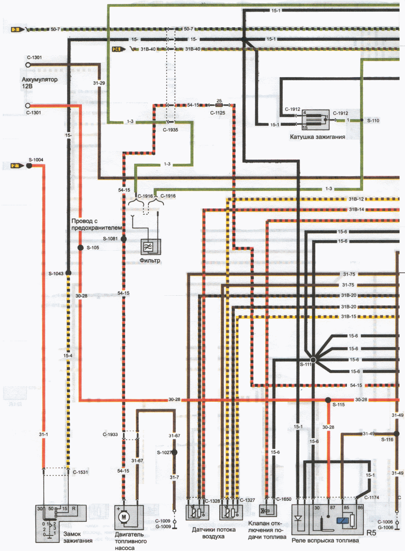
Схема электрического контура системы управления двигателем 2,8 дм 3
