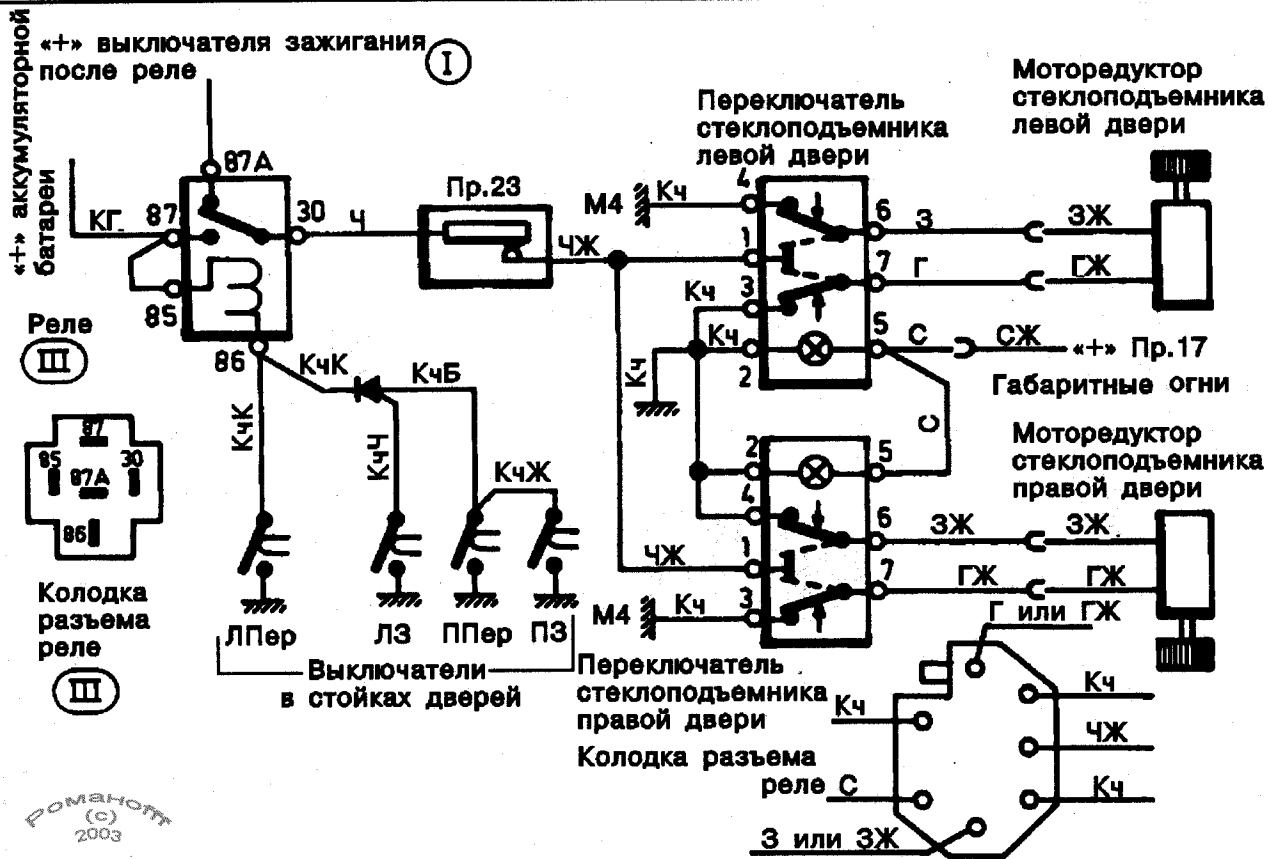
Схема включения стеклоподъемников передних дверей на модификациях «CL» и «GL»
