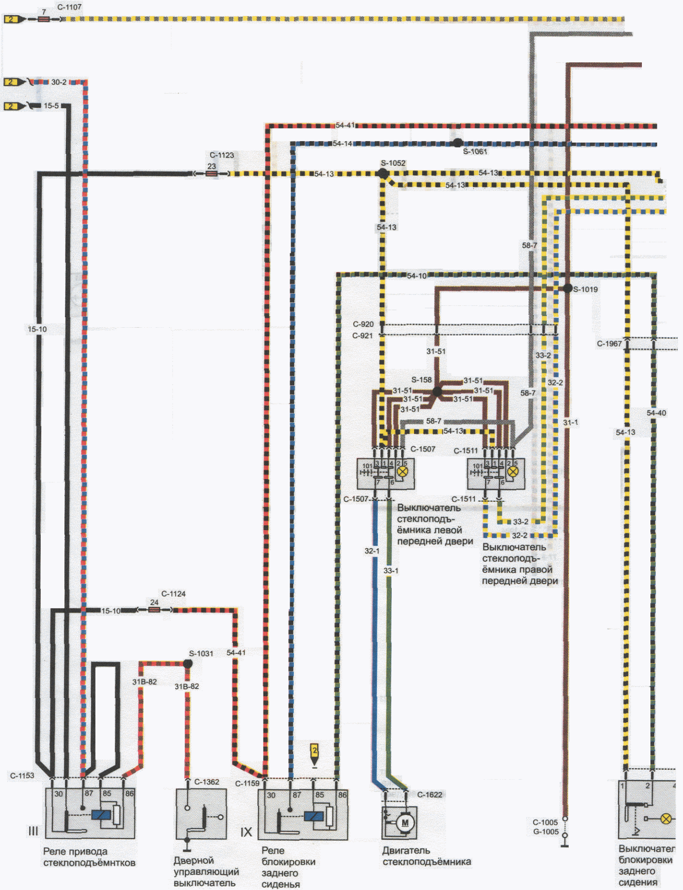
Схема электрического контура привода стеклоподъемника
