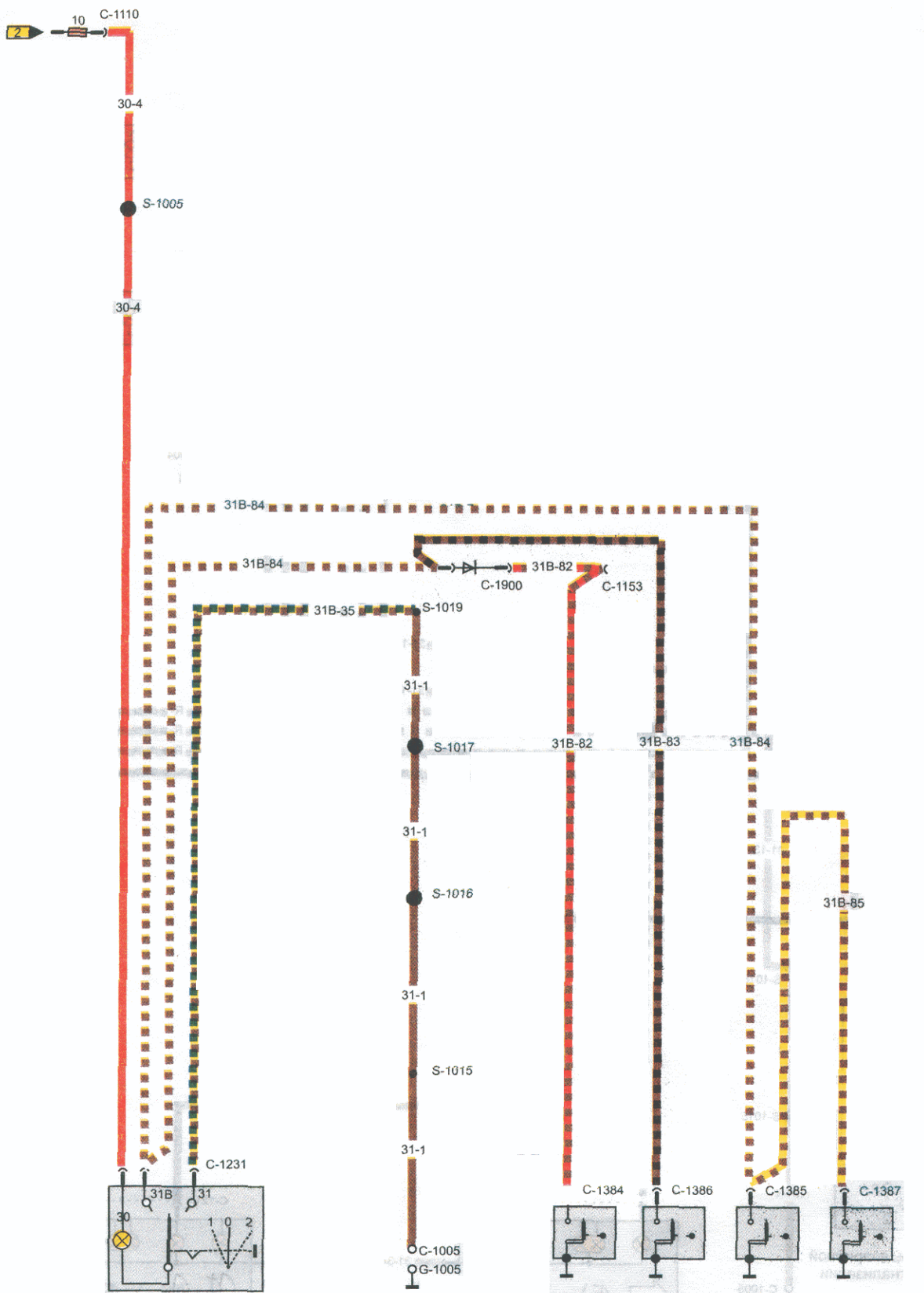
Дверные выключатели внутреннего освещения
