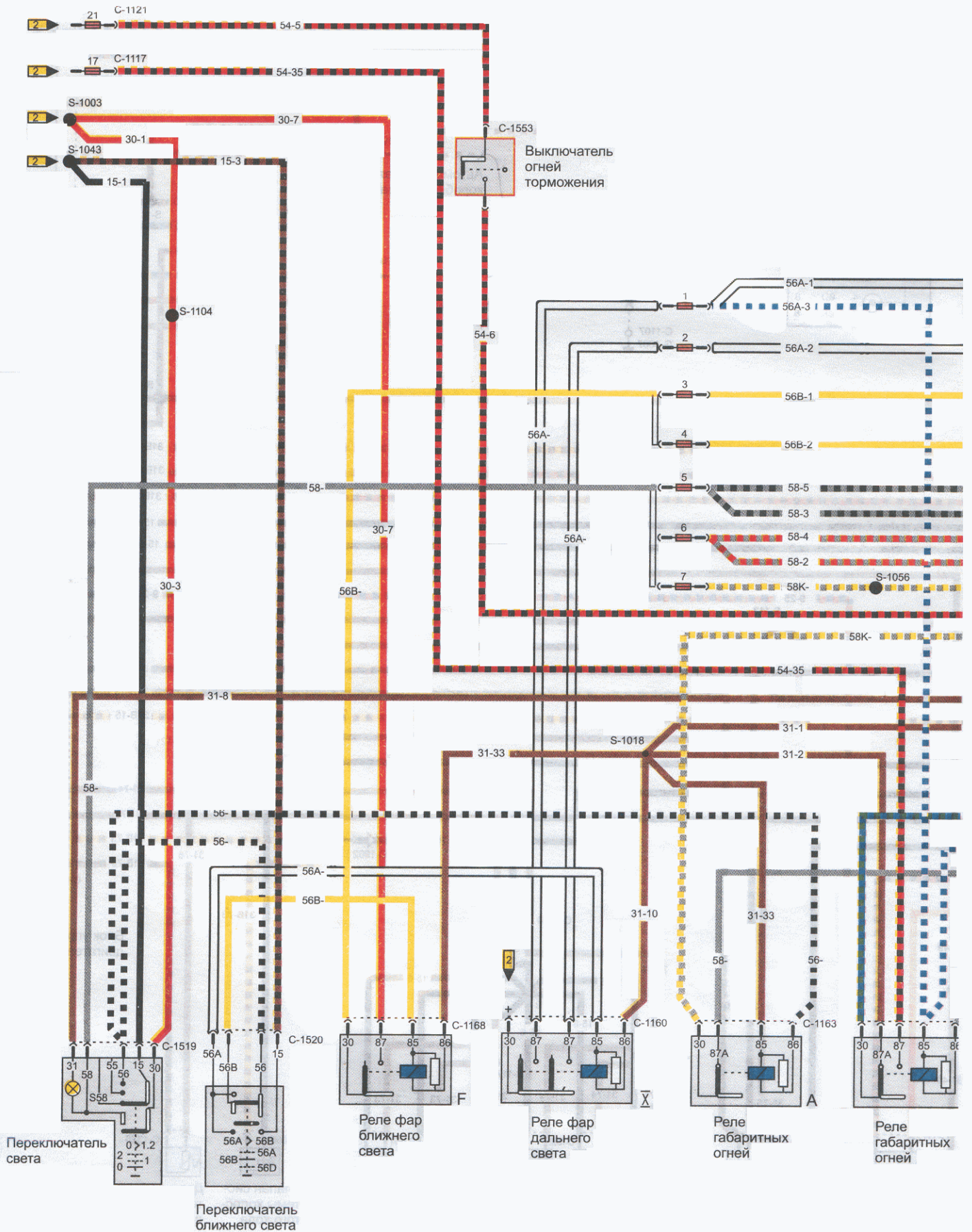
Схема электрического контура наружного освещения.
