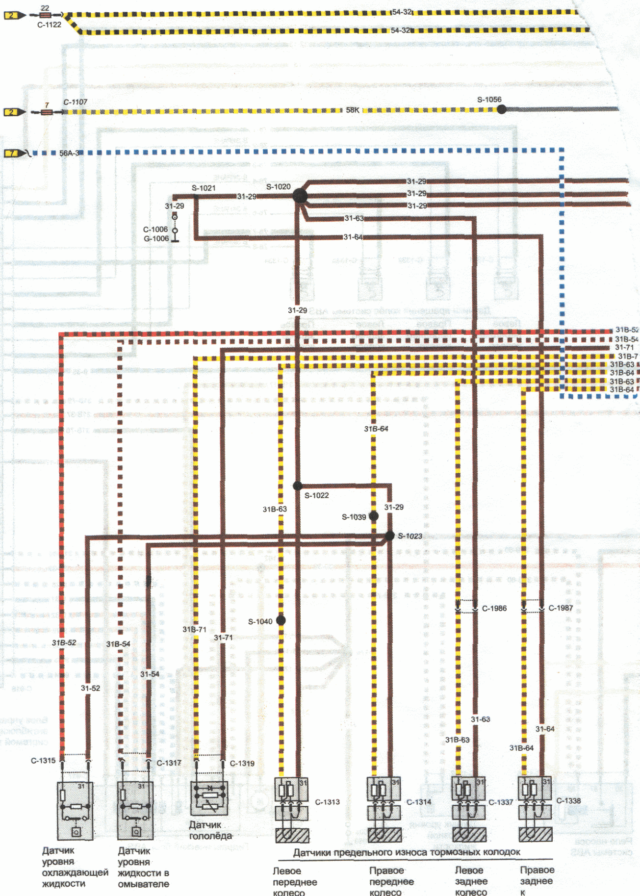
Схема электрического контура дополнительной контрольной системы AWS
