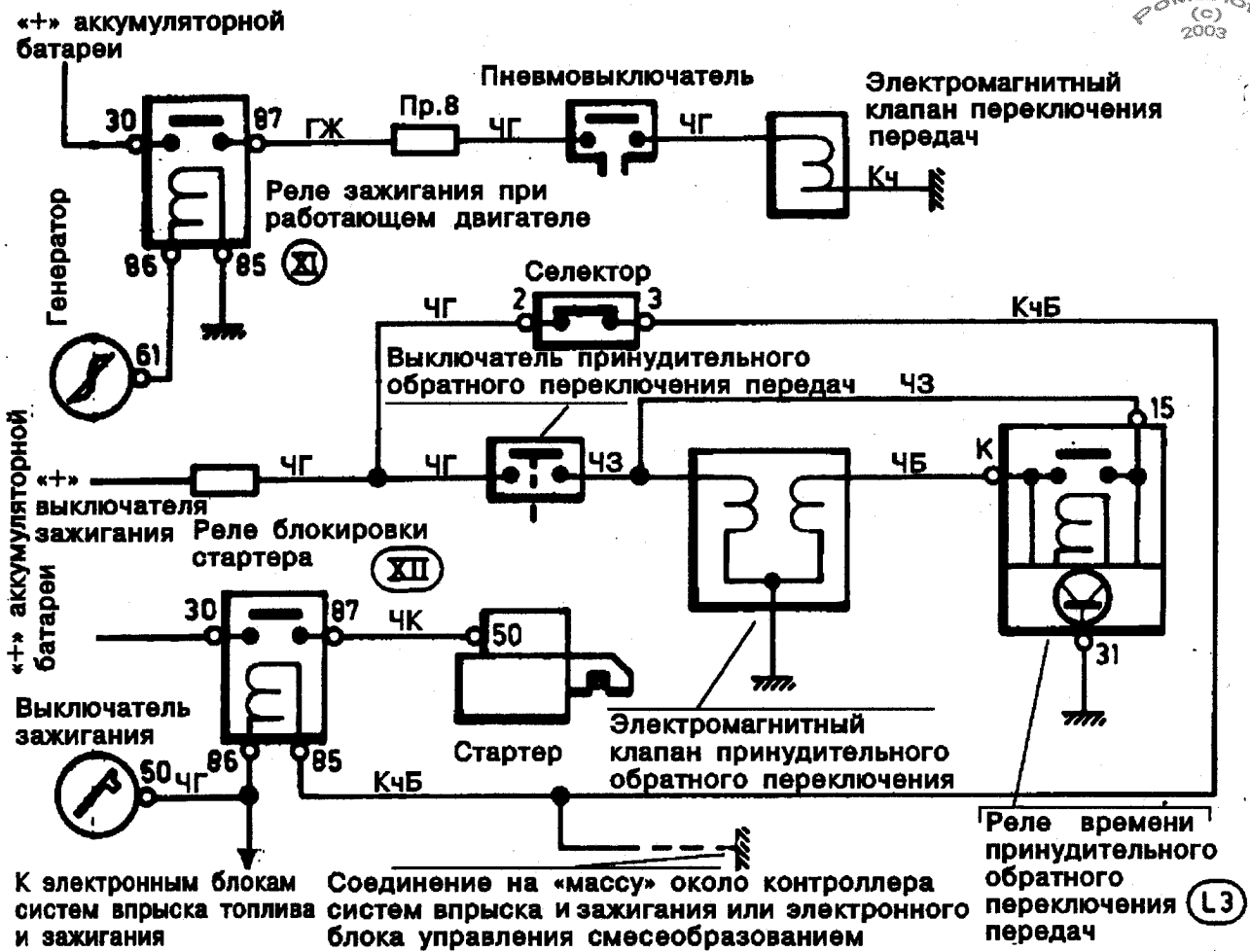
Схема включения электрических узлов автоматической трансмиссии
