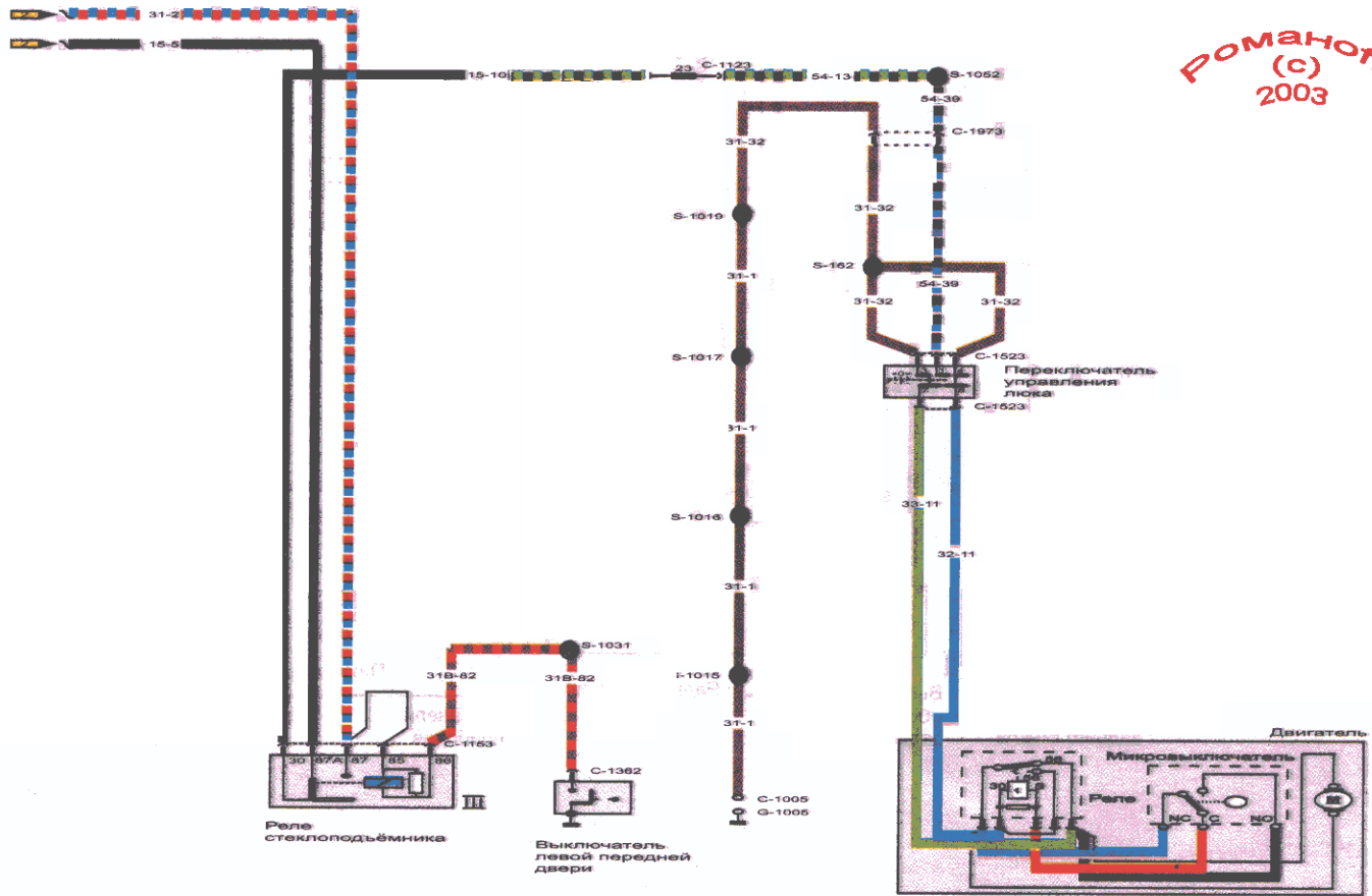
Схема электрического контура привода люка.
