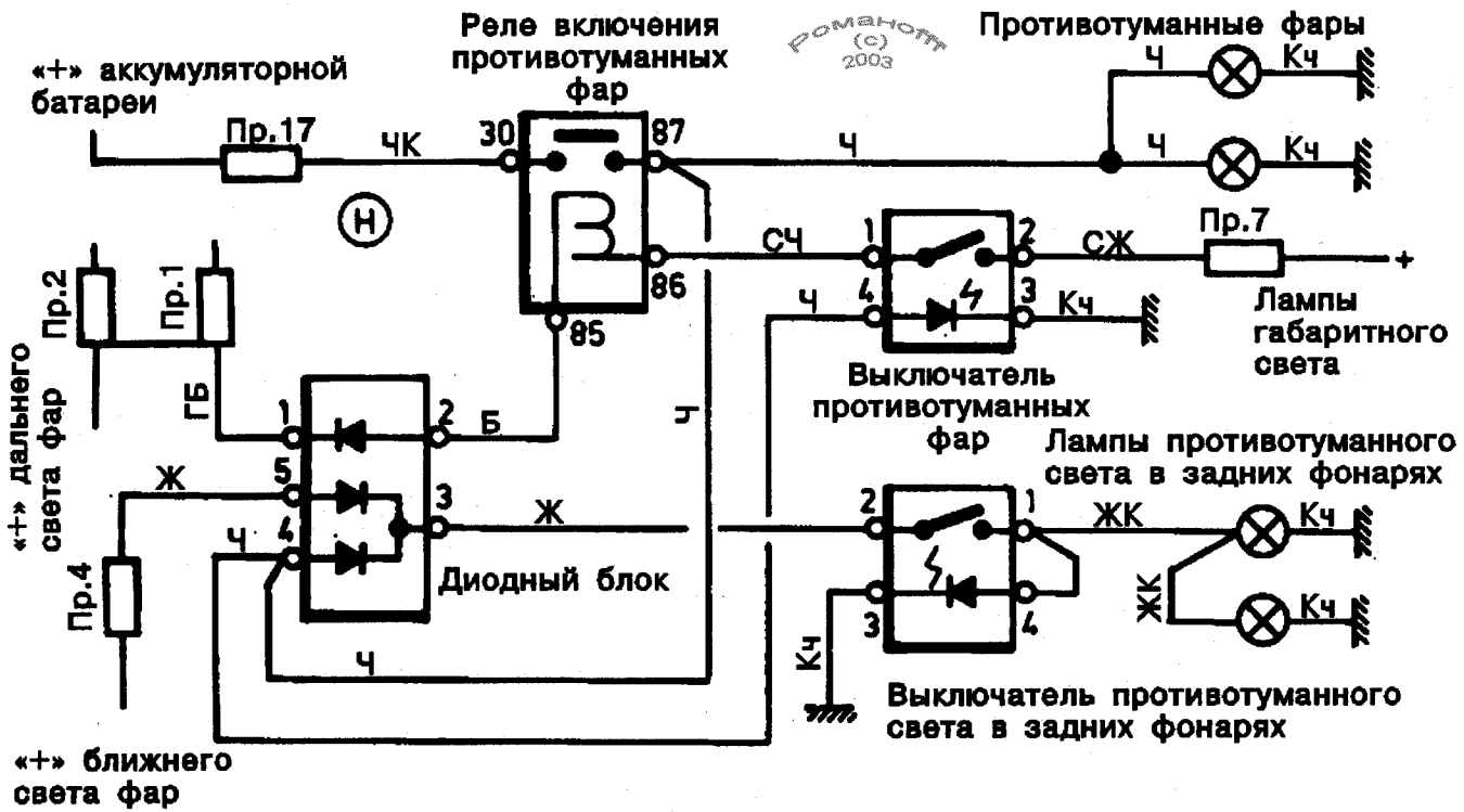
Схема включения противотуманных фар и противотуманного света в задних фонарях
