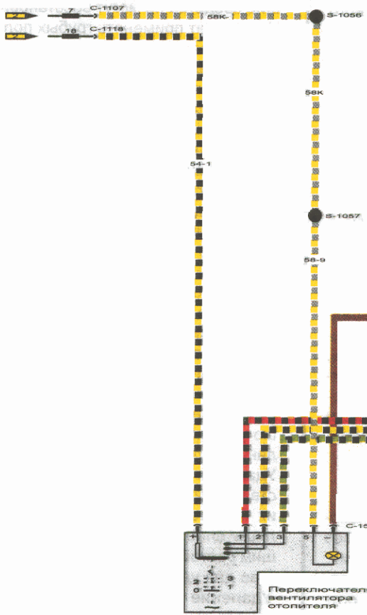
Схема электрического контура включения вентилятора отопителя.
